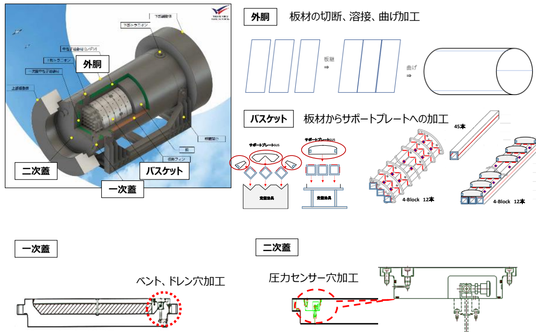
図 2：キャスク部品（例示）
